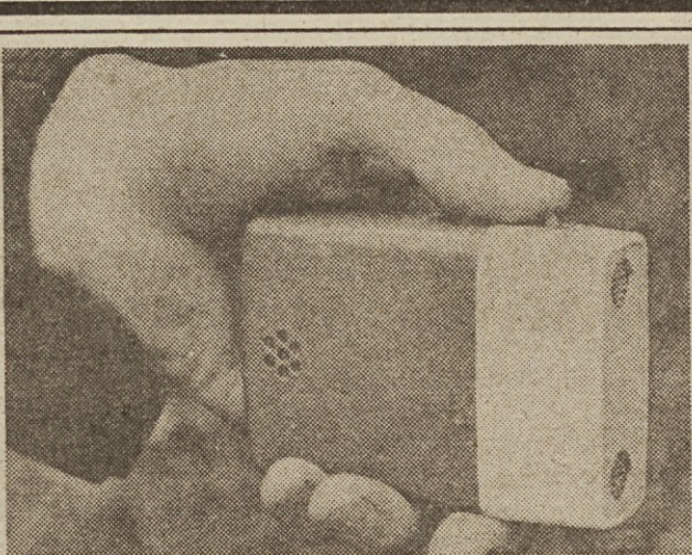
Poskusni ultrazvočni vodnik za slepe. Zvočni valovi, ki se odbijajo od ovire, se v majhnem sprejemniku spreminjajo v slišni signal ali pa začutiš brenčanje z dljanjo.
