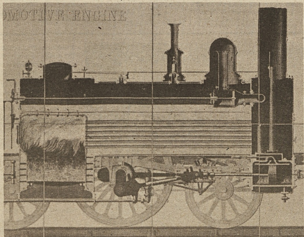
Stroj, ki je prinesel revolucijo v transport: tehnična risba parne lokomotive, 1848
