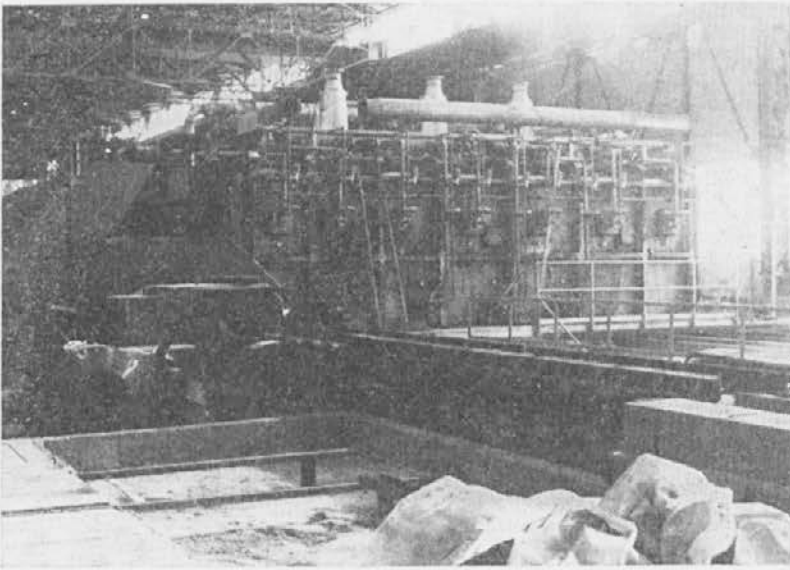
Hladilni tunel v končni fazi montaže z žago za vroče rezanje
