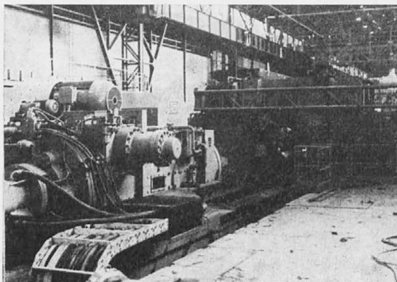
Vstopna stran kovaškega stroja
