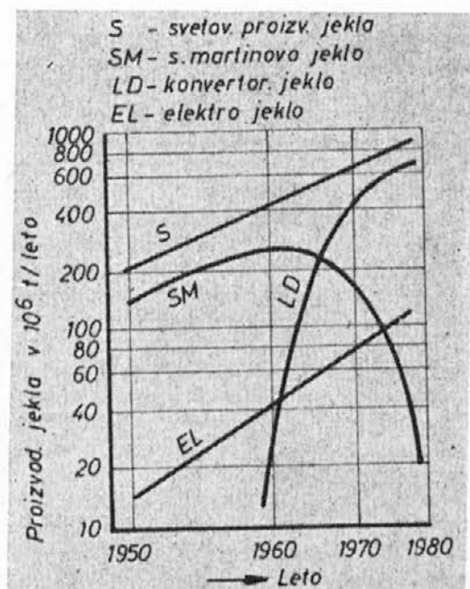
Diagram 1: Razvoj svetovne proizvodnje jekla, ločeno po postopkih
