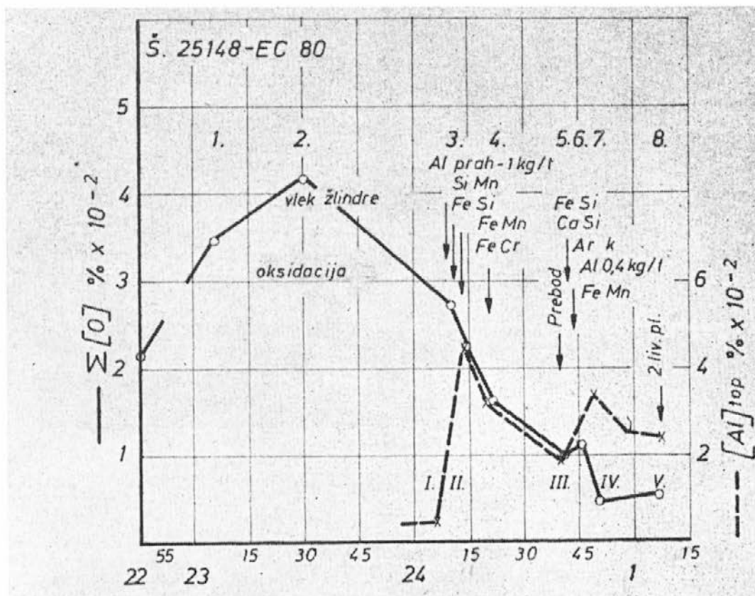
Diagram 42. Izdelava šarže 25148 kval. EC 80 z uporabo praš. dezoksidantov
