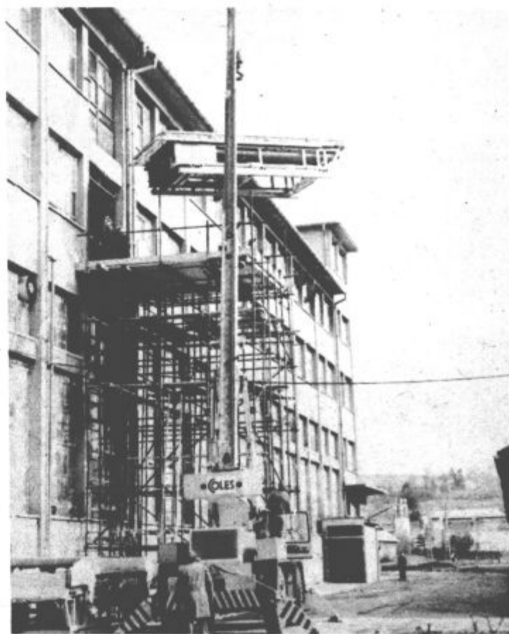
NAJVEČJI VAKUMSKI SUŠILNIK PRI NAS – V sredo, 2. novembra so v oddelek dodelave šoštanjske tovarne usnja pripeljali vakumski sušilnik, ki je največji v Jugoslaviji. Nabavili so ga v zvezi s preusmeritvijo proizvodnega programa v tozdu Tovarna usnja Šoštanj. Velikost ene sušilne plošče znaša 2,5 krat 6 metrov, zato so zaradi takih dimenzij sušilnik, čigar skupna teža znaša 9700 kilogramov, transportirali v dveh delih.
