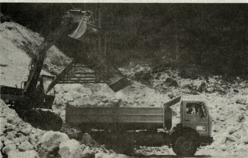
Poenostavljeno odbiranje prevelikih komadov iz posipnega materiala za gozdne ceste. - Foto GG
