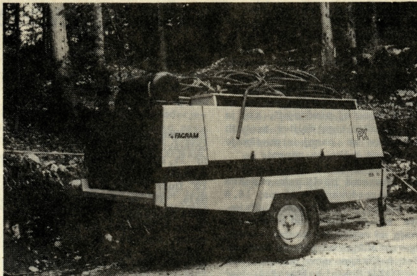
Nova izvedba kopresorja pri gradnji gozdnih cest na Jelovici Foto GG
