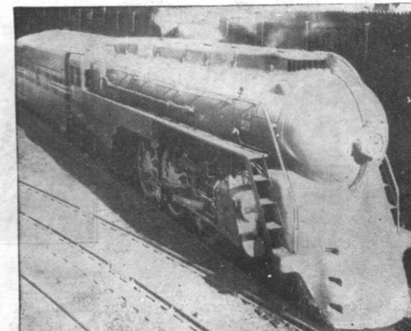
NAD 120 KM NA URO. Na progi New York—Chicago so uvedli nove aerodinamične motorne vlake tipa Hudson, ki vozijo z brzino nad 120 km na uro. Lokomotive imajo motorje po 4700 konjskih sil
