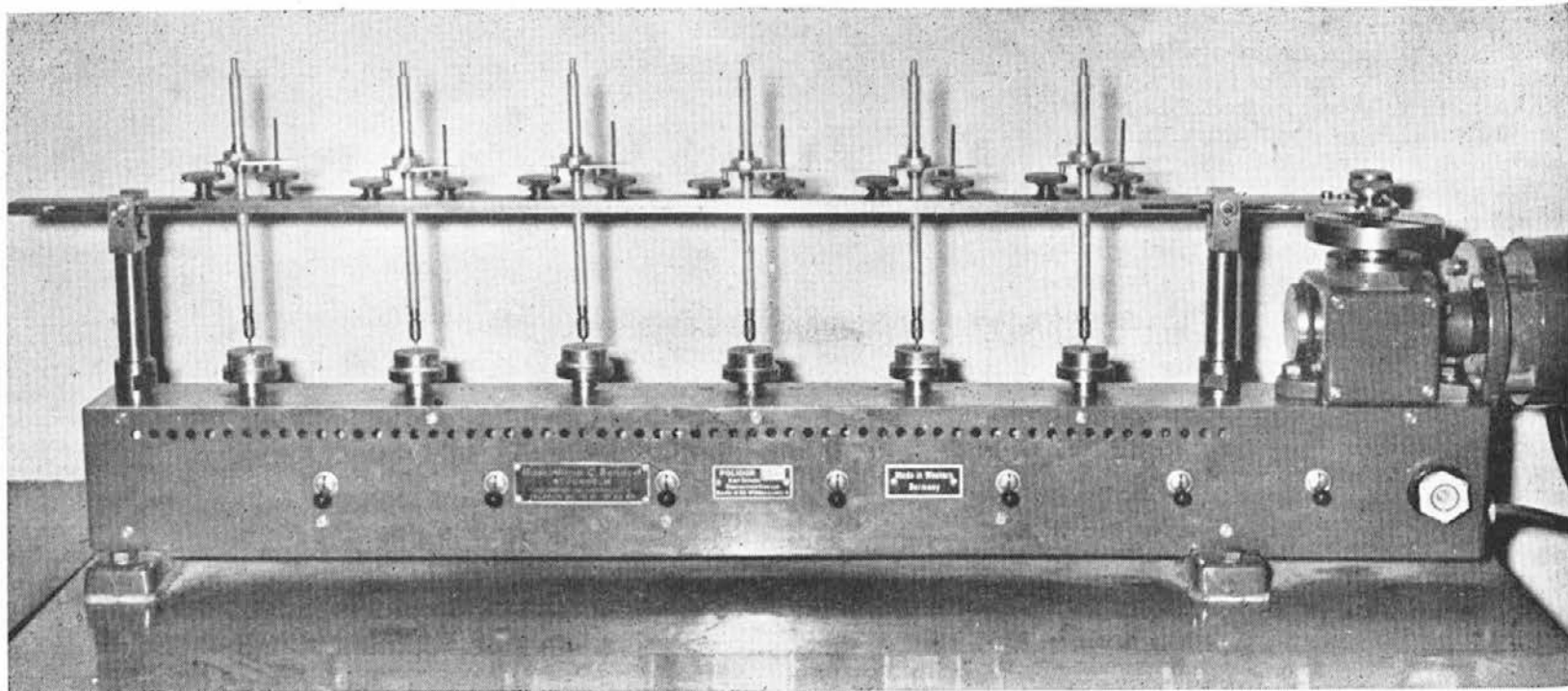
Naprava za poliranje diamantnih votlic. Da, izdelava grelne žice zahteva najbolj precizne in žlahtne operacije
