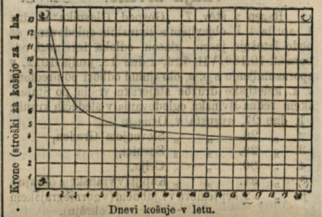
Stroškovni diagram kosilnega stroja, ako pokosi na dan 4 ha.
