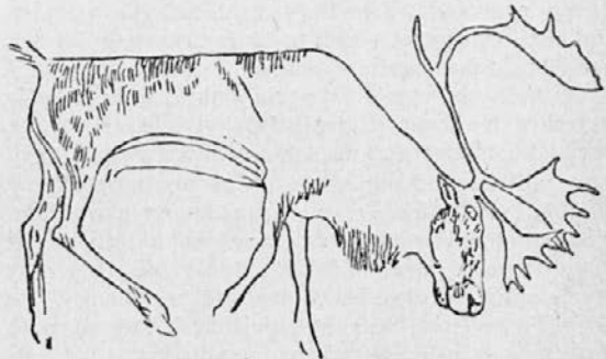
Severni jelen na paši. (Vrezana risba na kosu rogovja severnega jelena, ki so ga naši prapradedi nosili okoli vratu, da bi jim prinašal srečo na lovu.)
