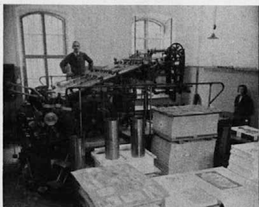
V strojnici za bakrotisk
