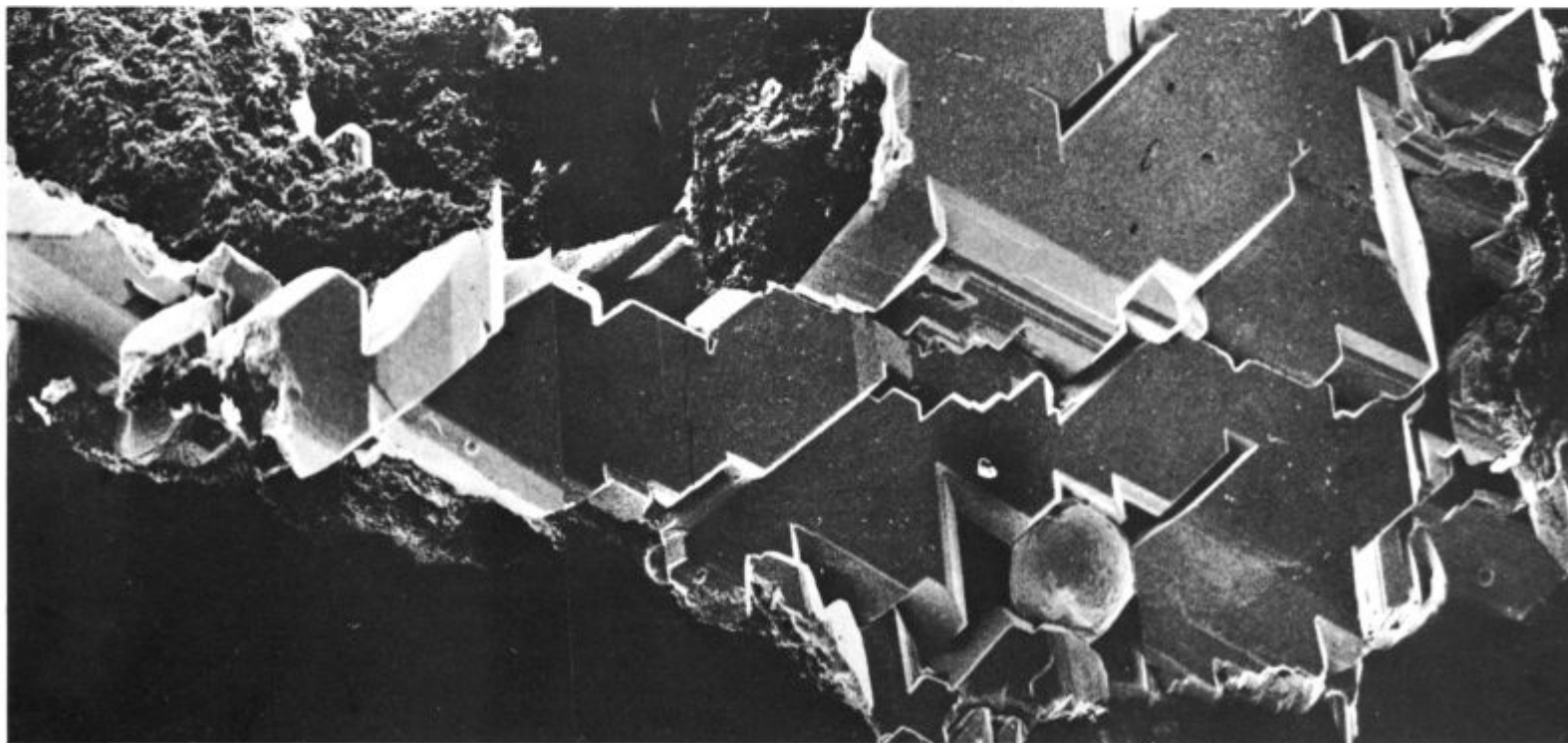
Kristalni ustroj cinabarita z vkleščeno »kapljo« živega srebra (posnetek z elektronskim mikroskopom, FNT, oddelek za montanistiko, foto Vlado Segalla)
