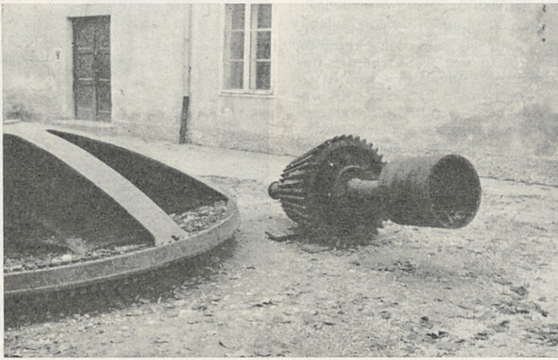
Multiplikator dotrajanega fužinskega vodnega agregata za pridobivanje električne energije iz leta 1922 je imel vgrajene lesene zobe; na dvorišču fužinskega gradu čaka na prevoz v muzej
