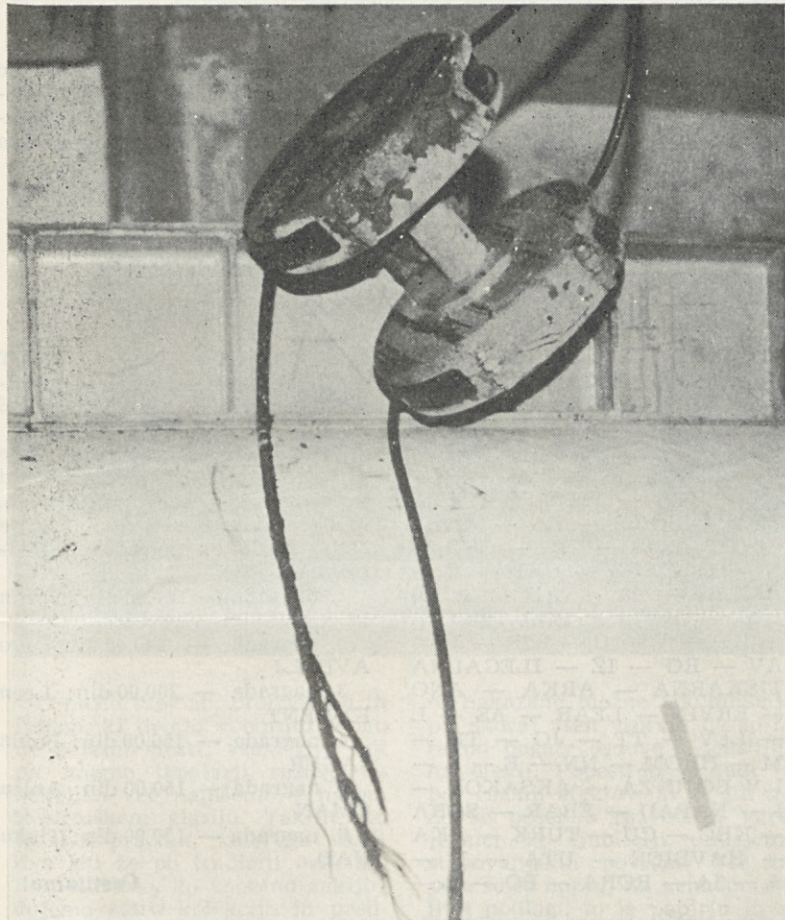
Kako se le lahko jeklena vrv dvigala takole razcefra, ko pa je bila dan ali dva pred tem atestirana?
