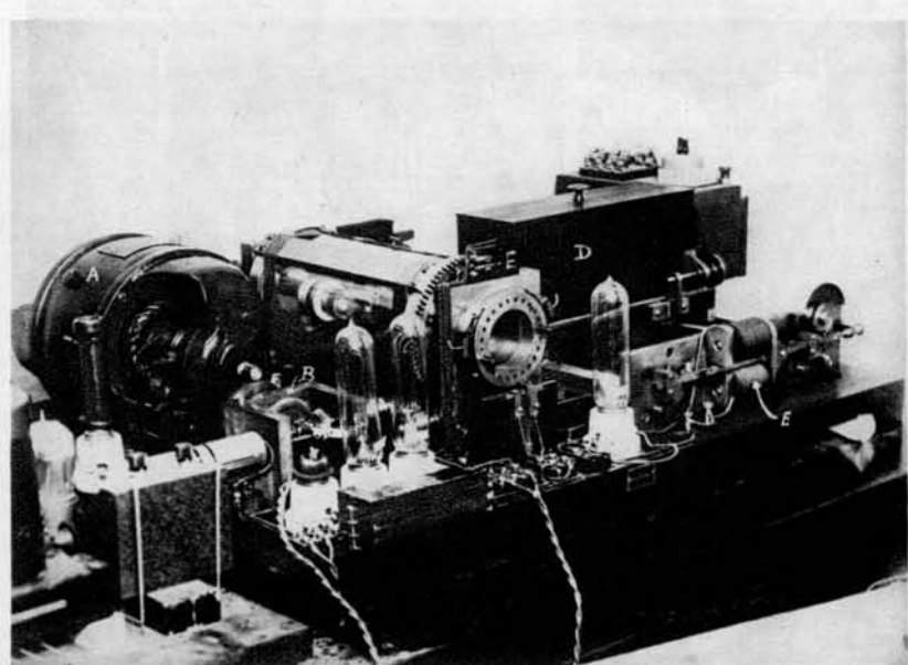
Brezžično prenašanje slik: pošiljalni aparat s kamero (D), ki sprejme poslano sliko
