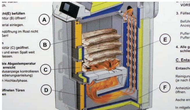
Nazorna predstavitev tega, kar se dogaja v peči.
