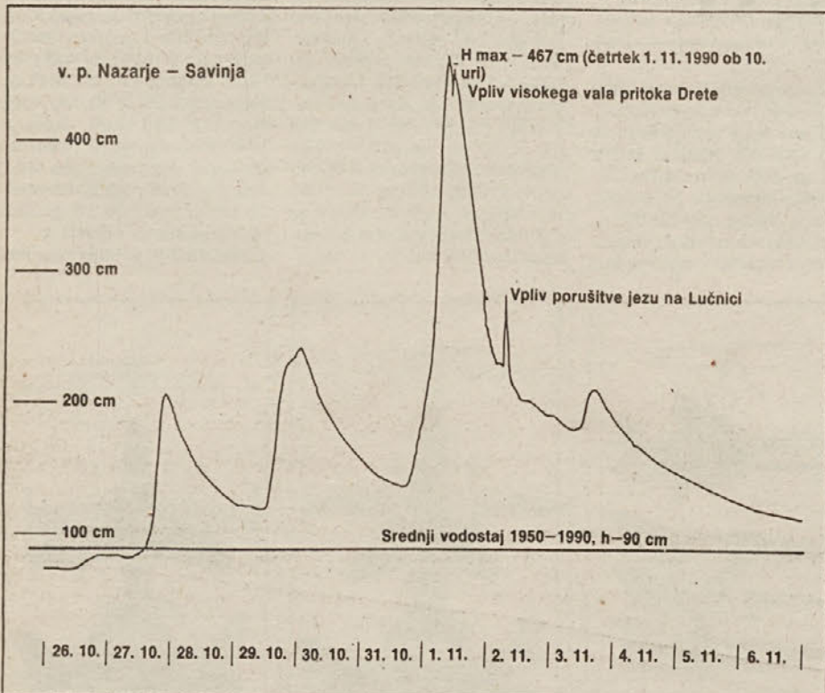
Nivogram vodomerne postaje Nazarje prikazuje potek gladine Savinje od 26. 10. 1990 do 6. 11. 1990
