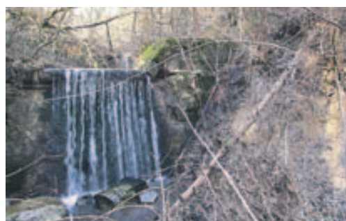
Ob zadnjih poplavih oktobra 2014 je hudourni voda prek teh zadrževalnikov odnesla velike količine prodnega materiala, katerega grobe frakcije so skoraj zasule strugo pri Gaberju (glej sliko), drobne frakcije pa je odnesla Gradaščica (naplavine so tudi že v Malem grabnu). V primeru porušitve teh zadrževalnikov bi proti Gradaščici odneslo skoraj 50.000 kubičnih metrov materiala.
