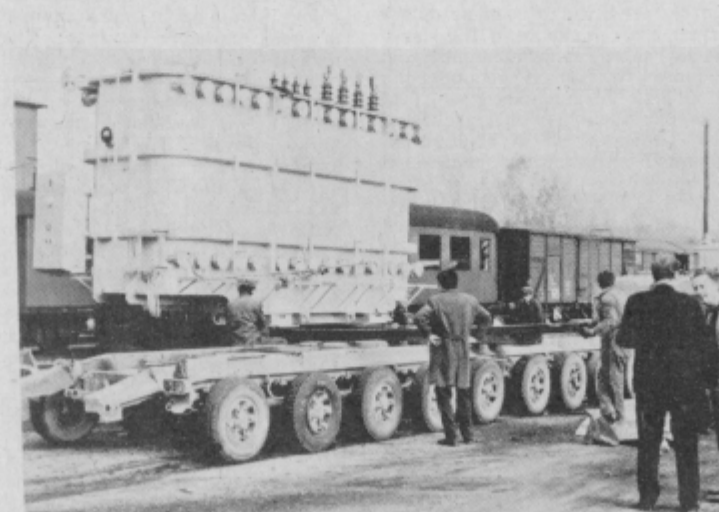
Transport 60 tonskega velikana iz vagona na cestno transportni vlačilec ni predstavljal delavcem Hidromontaže nobenega problema.
