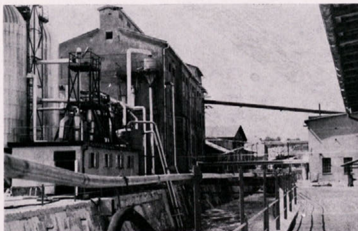
Pogled na kuharico celuloze. V ospredju levo je regeneracija SO 2 plina in toplote
