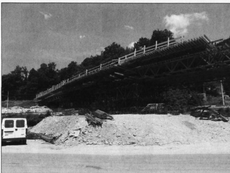
Gradnja nadvoza čez železnico pri Orehovem
