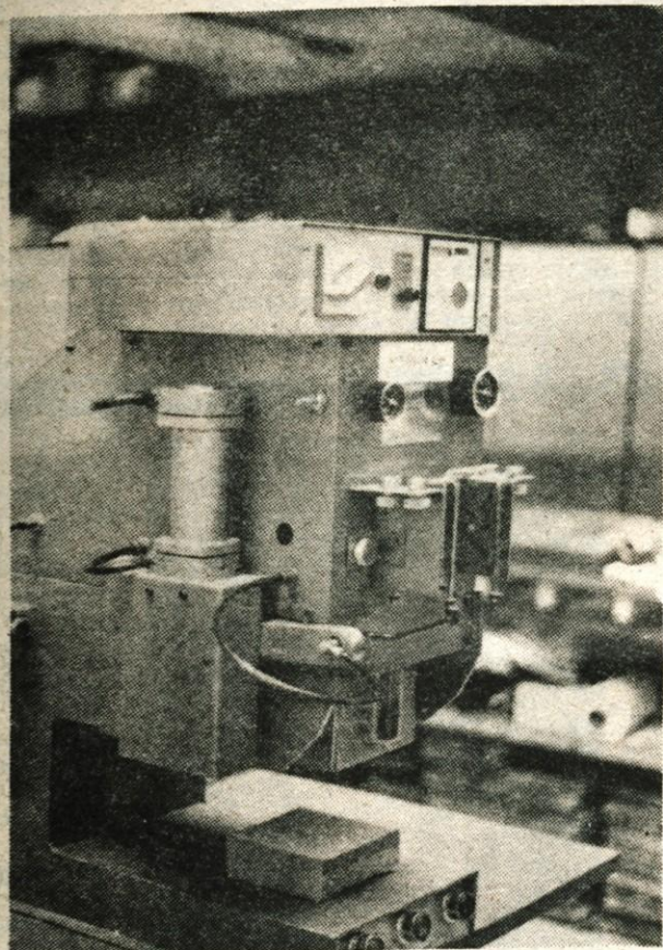
Novi stroj ETIPRES B 81, ki so ga naredili strokovnjaki v sodelovanju s Kladivarjem.
