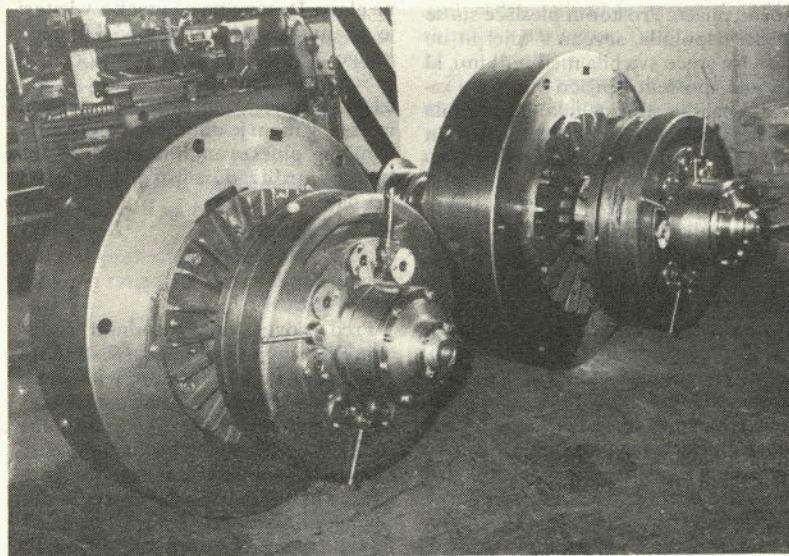
Sklopke z zavoro DA 315 izdelane v TOZD MO kot sestavni del težkih stiskalnic, ki jih izdeluje Metalna Maribor (foto Arzenšek)
