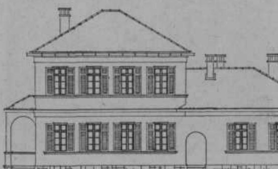
Tip školske zgrade sa 2 odjeljenja.
