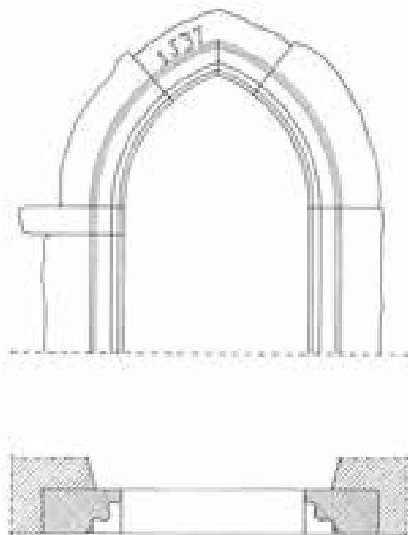
Izris dokumentiranega poznogotskega portala na glavni fasadi grajskega jedra. Pogled in tloris. Poskus rekonstrukcije na osnovi fotografije Cirila Velepčiča iz leta 1947 in skice Ivana Komelja iz leta 1949 (risal: Igor Sapač, 2003).
