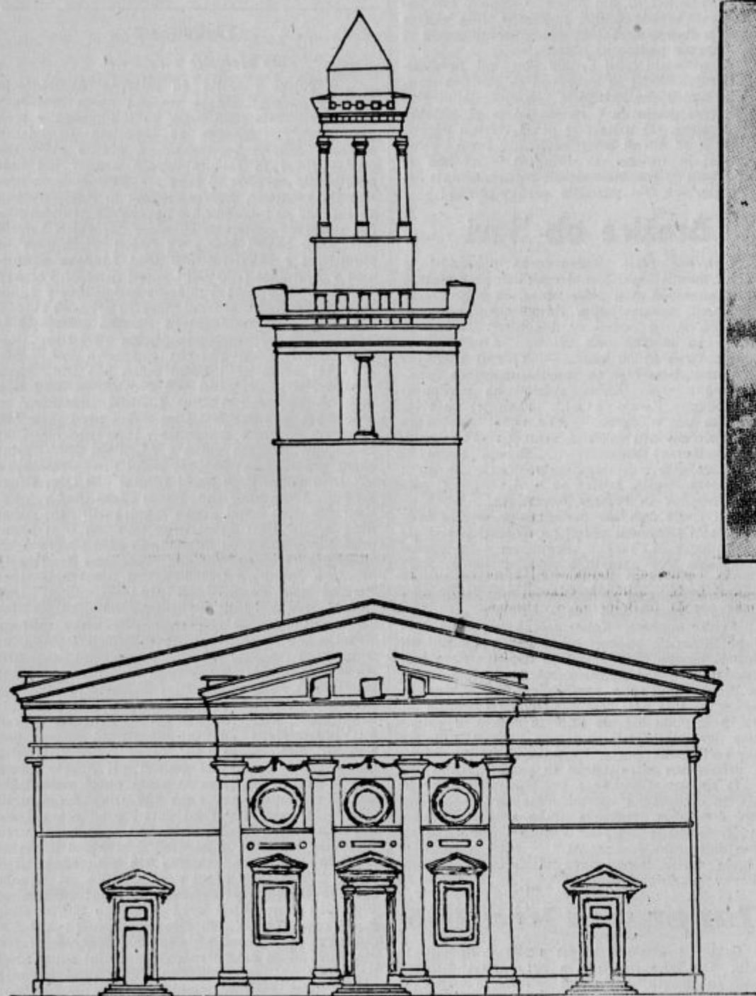
Načrt fasade nove frančiškanske cerkve v Šiški. — Izdelal naš arhitekt g. J. Plečnik.
