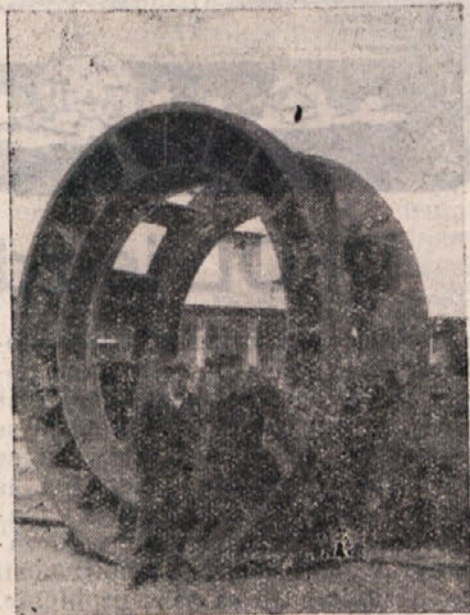
Kaplanova turbina — eden največjih odlitkov Litostroja
