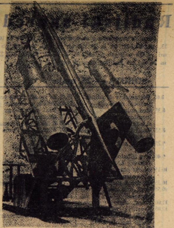
Dirigirano letalo na cilj C141, ki je opremljeno z dvema reaktivnima motorjema in ga izstrelijo s posebne naprave. V 80 sekundah doseže višino 20.000 metrov.
