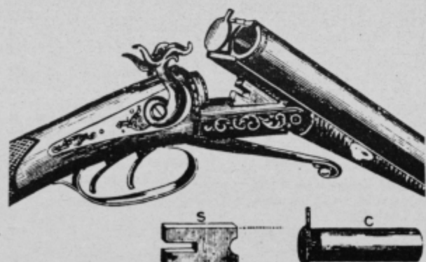
Dvocevna prelamača Lefauchaux
