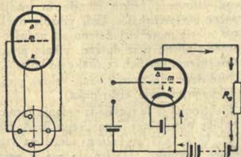
Levo: Trioda in njen podstavek. — Desno: Principialna vezava triode. Naznačen je tir elektronov.
