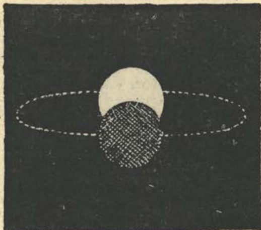
Binarni sistem. Zvezda Algol s svojim temnim spremeljalcem. To ni fotografija, temveč risba po znanstvenih ugotovitvah.
