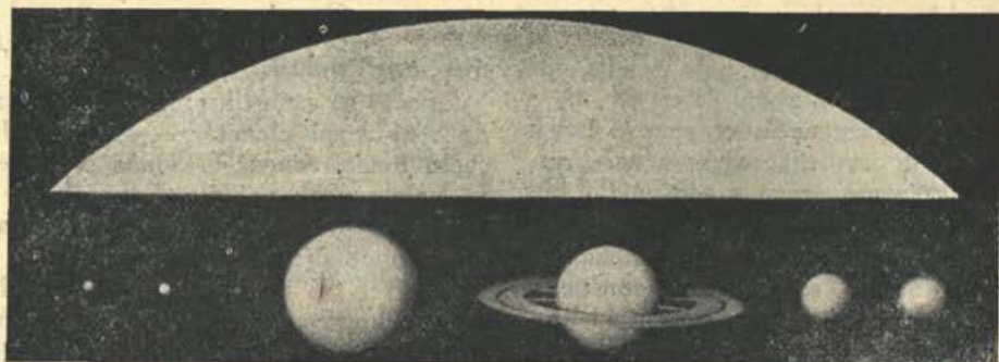
Relativne velikosti sonca in planetov. Planeti so razvrščeni tako, da je na skrajni levici Merkur, ki mu sledi Venera, potem je zemlja z luno, dalje Mars, potem velikan Jupiter, Saturn s svojim obročem, Uran, Neptun in kot zadnji Pluton. Od sonca je naslikan samo krajec. Razdalje seveda ne ustrezajo resničnemu stanju.
