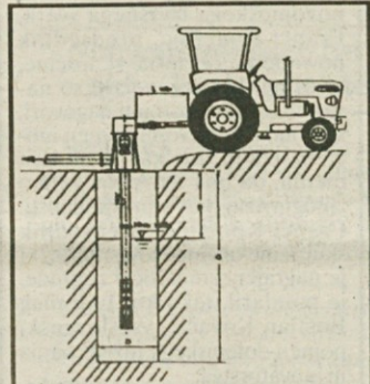
POMAGAJ SI SAM - Namakanje s pomočjo Litostrojeve črpalke.
