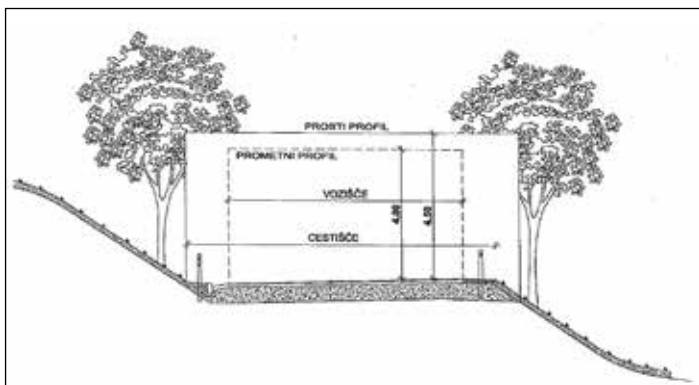
Primer prometnega profila (potrebna širina in višina sečnje)
