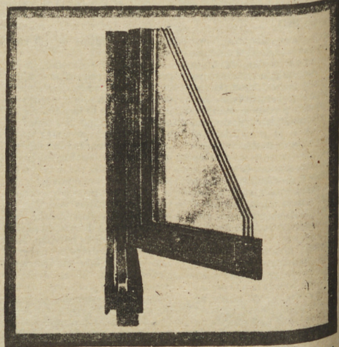
OKNO IZOPLUS ZASTEKLJENO S TRISLOJNIM IZO STEKLOM — PREREZ
