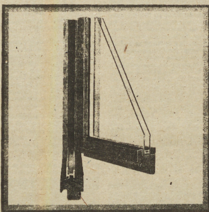
OKNO ZASTEKLJENO Z DVOSLOJNIM IZO STEKLOM — PREREZ
