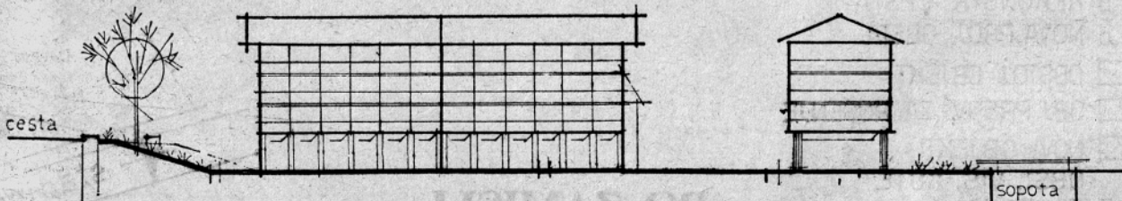
CENTER RADEČE PO IDEJNI ZASNOVI V PREREZU SMER SEVER-JUG (B-B)
