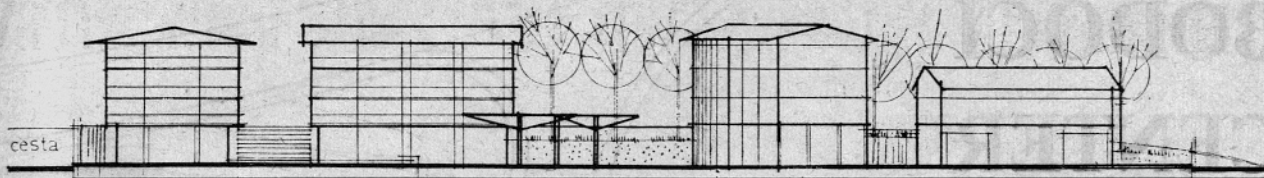
CENTER RADEČE PO IDEJNI ZASNOVI V PREREZU SMER VZHOD-ZAHOD (A-A)
