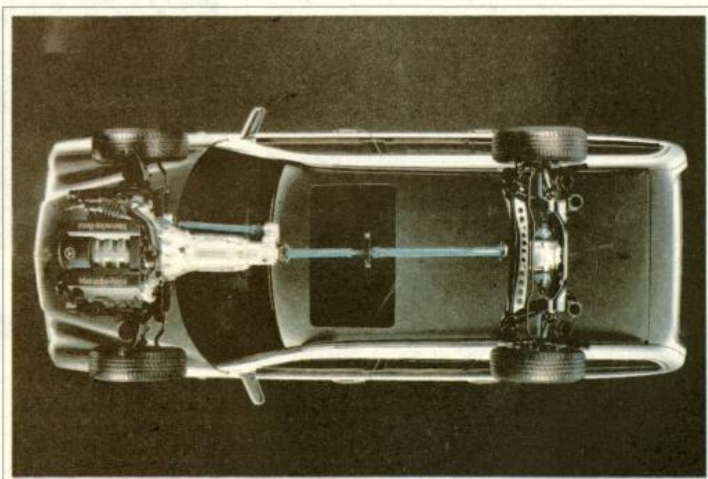
Shema 4Matic pogona pri Mercedes Benzu.
