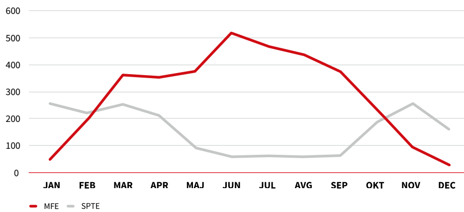
Proizvedena količina električne energije (v MWh) v MFE in SPTE po mesecih leta 2021
