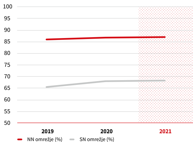
Delež omrežja v kabelski izvedbi od leta 2019 do leta 2021
