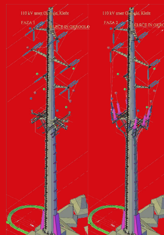
3D-model poligonalnega cevnega stebra, tehnična rešitev zaposlenih
