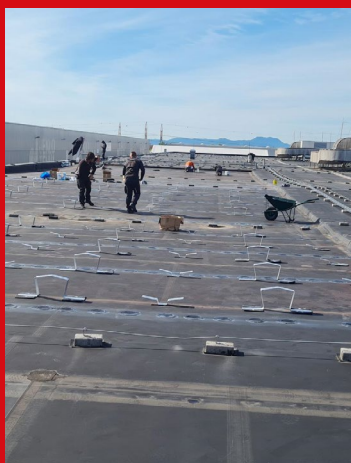
Gradnja sončne elektrarne na strehi trgovskega centra
