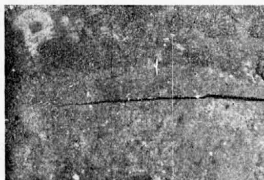
Slika 3 — napetostna razpoka na ingotu
