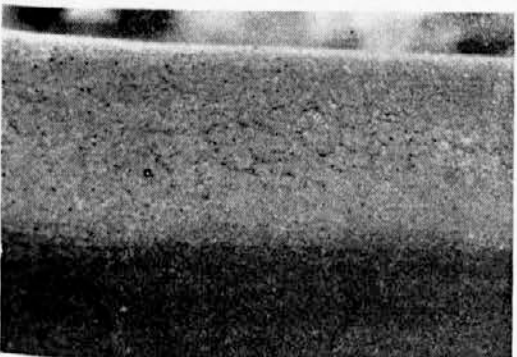
Slika 8 — mrežasta površina ingota
