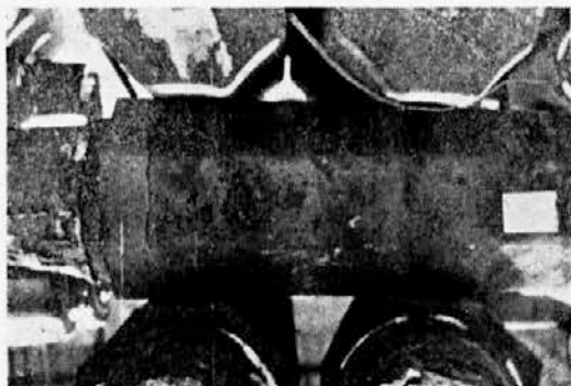
Slika 1 — vroča prečna razpoka na ingotu C 1121
