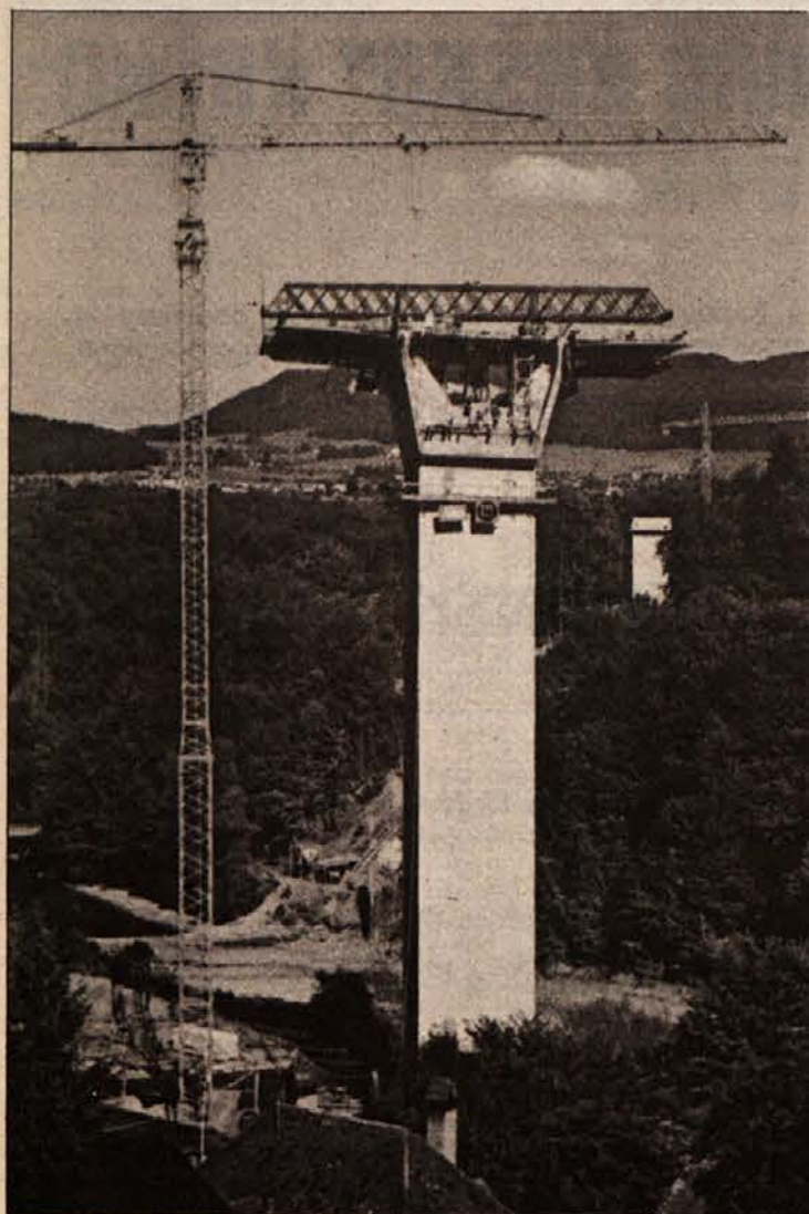
Vrtljivi stolpni žerjav LM 90.1 HC
