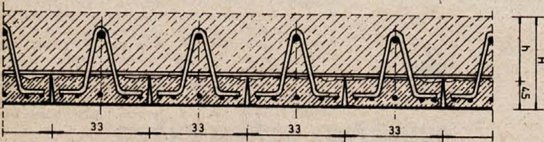
PREČNI PREREZ SKOZI STROP
