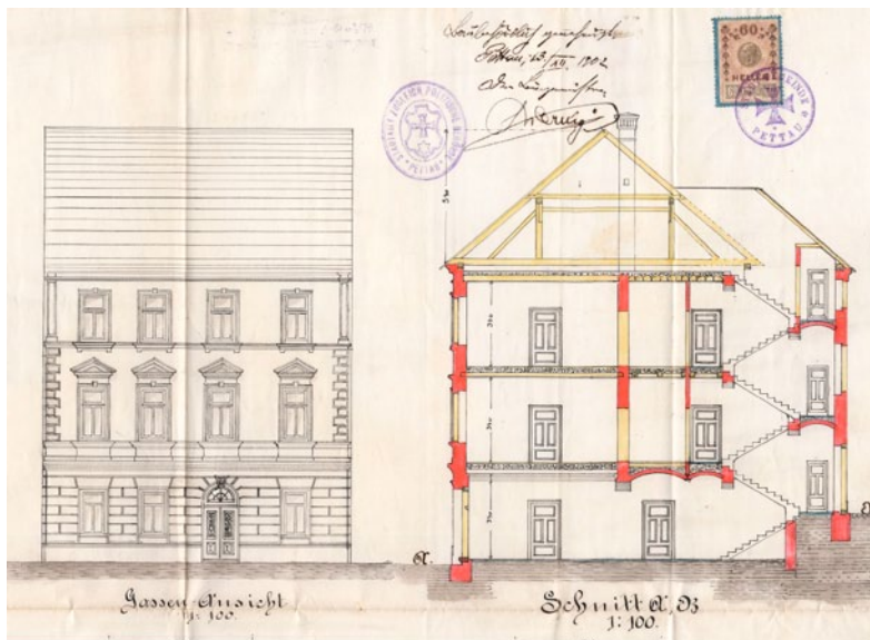
Načrt prenove hiše Antona Neubauerja (pročelje, prerez), 1901
