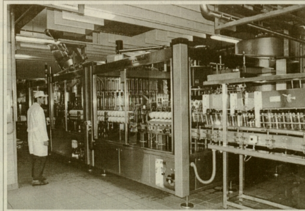
Zmogljivost nove polnilne linije za vodo, ki je stala okrog ene milijarde tolarjev, je 12 tisoč 1,5-litrskih steklenic na uro. Linija, ki je energetska varčna in tudi okolju prijazna, je prirejena za polnjenje plastenk od 0,25 do 2,5 litra in steklenic od 0,25 do 0,5 litra.
