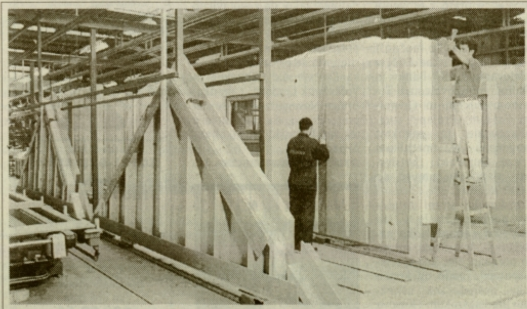
Finalna obdelava zunanjih stenskih elementov v Preddvoru.
