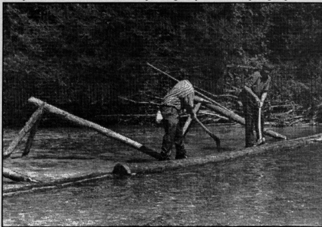
Prikaz plavljenja lesa po Savinji
