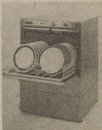
Pomivalni stroj PS-70/1, ki ga je razvil ing. Kadunc Dušan s sodelavci. Za ta stroj so dali tudi modelno prijavo zveznemu Zavodu za patente.
