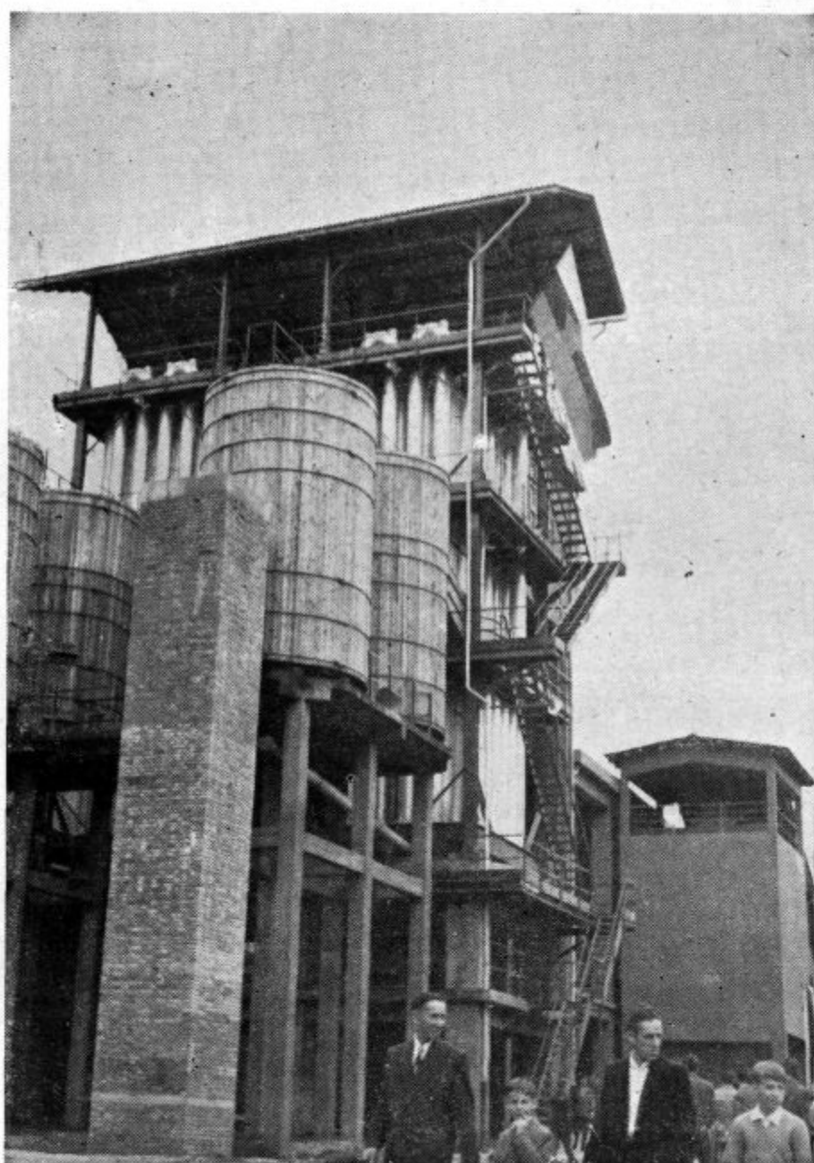
Nova rotacijska peč
