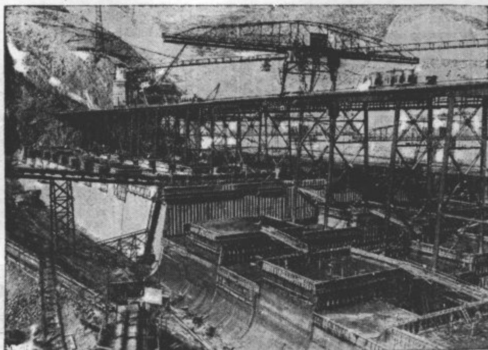
VELEDELO MODERNE TEHNIKE. V državi Washington (USA) dovršujejo največjo dolinsko pregrado na svetu
