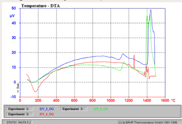
152 Ogrevne DTA krivulje vzorcev DV-3, DV-4 in DV-5
