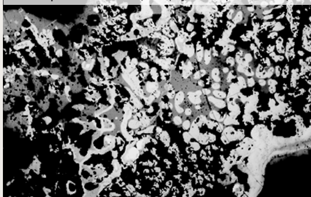
145 Mikroposnetek vzorca DV-3 (fajalit-olivin)
