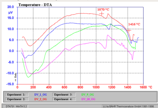
151 Ogrevne DTA krivulje vzorcev DV-1, DV-2, DV-9 in DV-10
