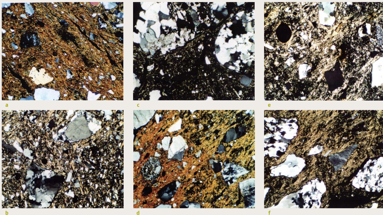
138 Mikrofotos von Dünnschliffen (alle Aufnahmen sind mit vollständig oder teilweise gekreuzten Polarisationsfiltern und mit gleicher Vergrößerung gemacht, die Bildbreite entspricht bei allen Abbildungen 2,5 mm):
