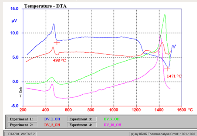
154 Ohlajevalne DTA krivulje vzorcev DV-1, DV-2, DV-9 in DV-10.
