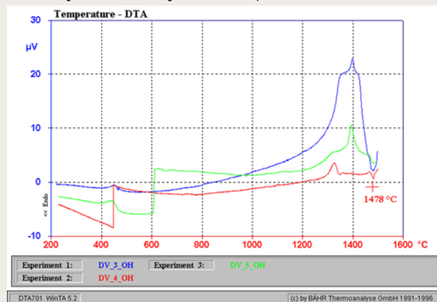
155 Ohlajevalne DTA krivulje vzorcev DV-3, DV-4 in DV-5.
