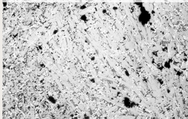
149 Majhni dendriti wüstita v fajalitni osnovi
