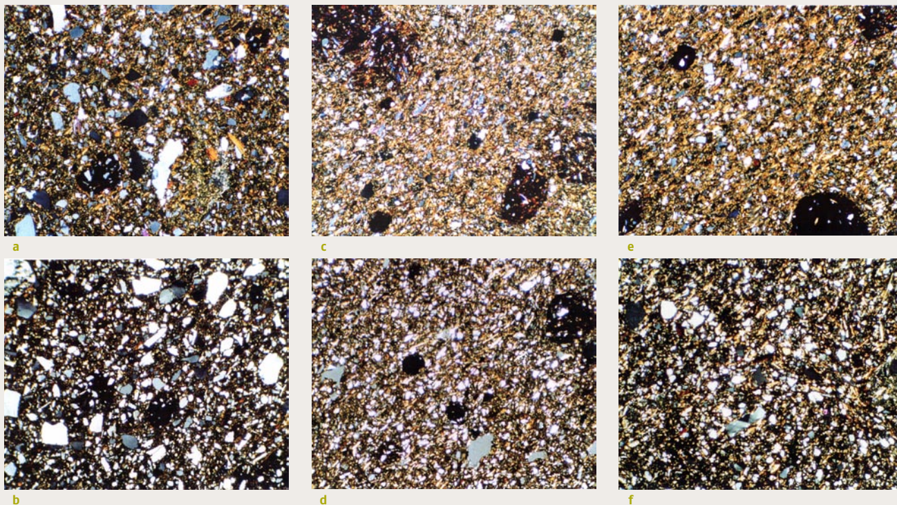
134 Mikrofotos von Dünnschliffen (alle Aufnahmen sind mit vollständig oder teilweise gekreuzten Polarisationsfiltern und mit gleicher Vergrößerung gemacht, die Bildbreite entspricht bei allen Abbildungen 2,5 mm):
