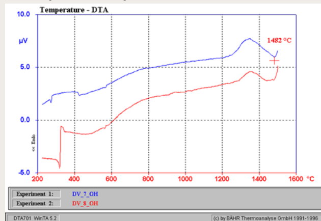
156 Ohlajevalne DTA krivulje vzorcev DV-7 in DV-8.
