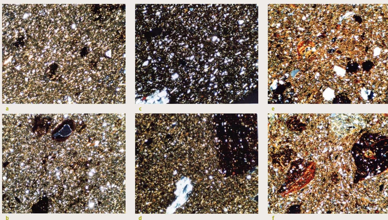
140 Mikrofotos von Dünnschliffen (alle Aufnahmen sind mit vollständig oder teilweise gekreuzten Polarisationsfiltern und mit gleicher Vergrößerung gemacht, die Bildbreite entspricht bei allen Abbildungen 2,5 mm):
