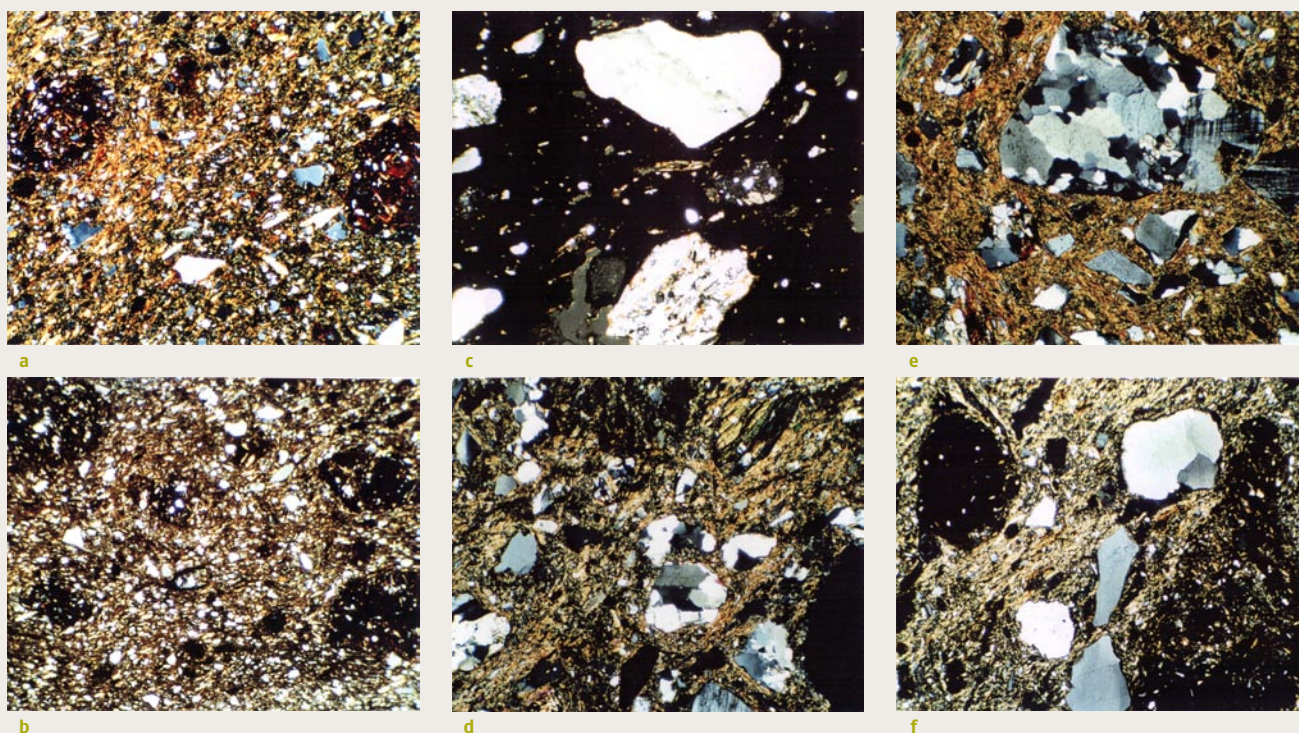
136 Mikrofotos von Dünnschliffen (alle Aufnahmen sind mit vollständig oder teilweise gekreuzten Polarisationsfiltern und mit gleicher Vergrößerung gemacht, die Bildbreite entspricht bei allen Abbildungen 2,5 mm):
