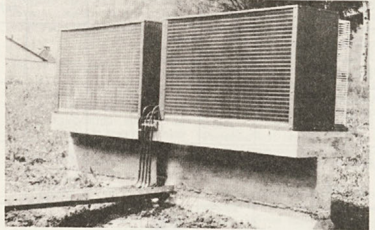
V minulem tednu je z dvomesečno zamudo začela obratovati klimatska naprava, ki vzdržuje ustrezno temperaturo in vlago v prostoru kjer se nahaja naš novi računalnik. Na zgornjem posnetku sta zračna kondenzatorja ki sta sestavni del klimatske naprave.
