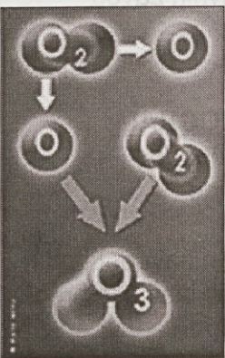
Sliki prikazujeta molekulo O 3
