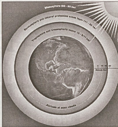
Ozon se nahaja v stratosferi in troposferi. Največjo gostoto doseže ozonski sloj pri višini 25 km.
