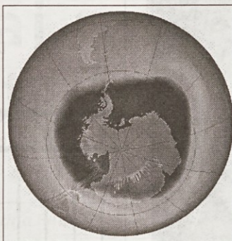
Velikost ozonske luknje, 7. 9.2007
