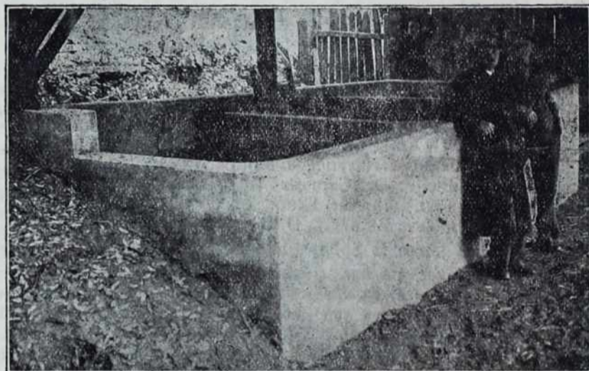
Kmetijski silos v D. Lendavi Mere posamezne jame so: 1,75 x 1,75 x 3,50 m.
