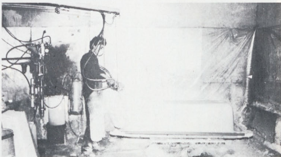
Armiranje kopalnih kadi s poliestrom
