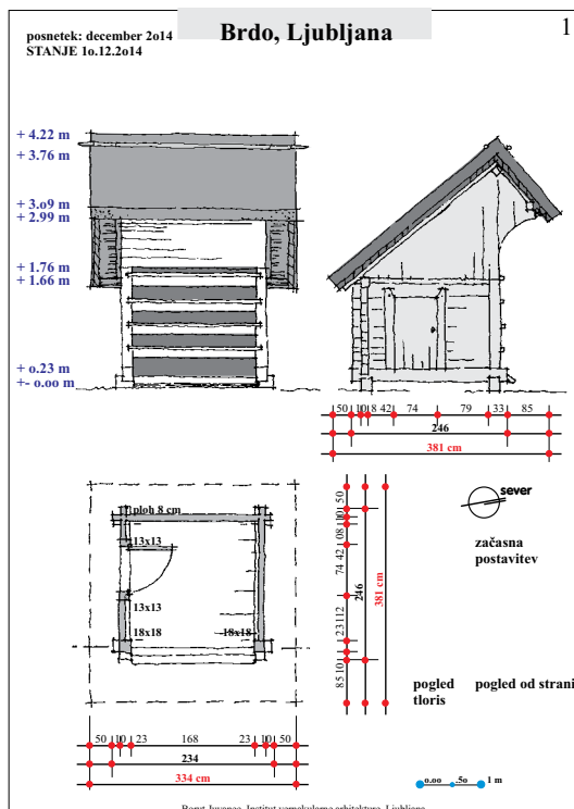
Tehnični načrti (tloris, prerez in pogled od spredaj) v merilu 1 : 50.
