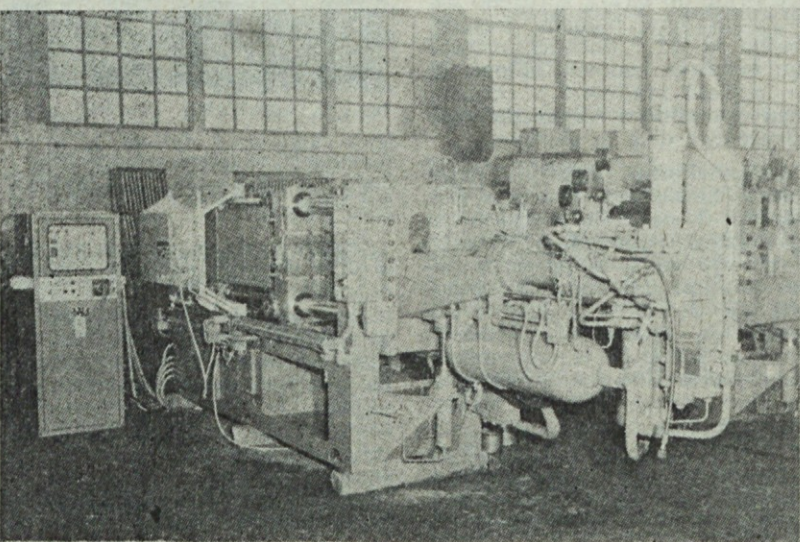
Že dokončan stroj za tlačno litje, ki smo ga izdelali za firmo WOTAN v ZRN (Foto J. J.)
