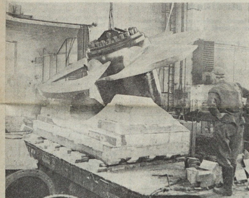
Nov petkrilni Kaplanov gonilnik za HE Dravograd pred transportom v elektrarno (Foto J. J.)
