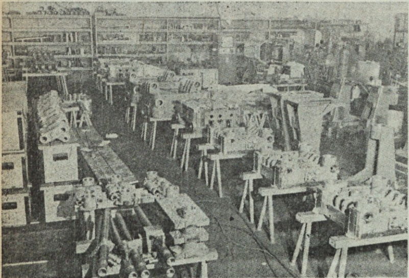
Pogled na pripravo sestavnih delov strojev za tlačno litje v montaži
