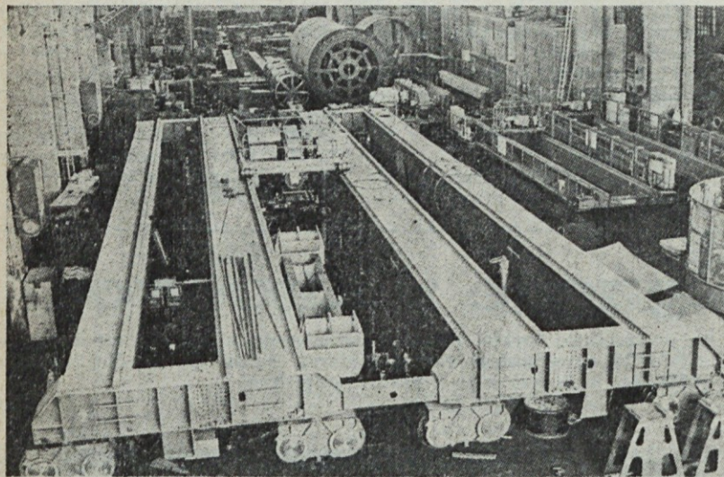
V juliju bomo odpremili električni mostovni tekalni žerjav za železarno Zawircie na Poljskem. (Tehnični podatki 180/32 Mp x 27,1 m)
