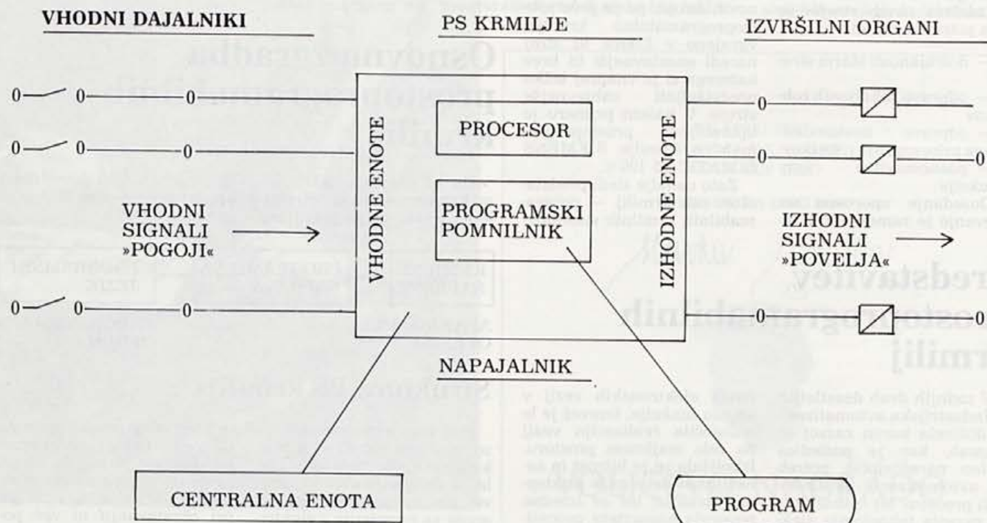
OSNOVNA ZGRADBA PS KRMILJA
