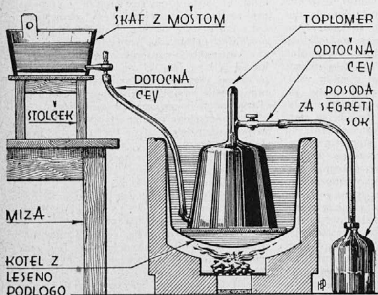
Zvonasti razgrevalnik-sterilizator v obratu
