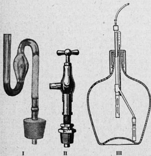
I Zračno cedilo z veho. Skozenj prihajajoči zrak je čist in ne okuži sladoseka. — II Kovinska pipa, skozi katero se pri točenju ne morejo zatositi v sladosek kvasnice. — III Električni sterilizator za steriliziranje sladoseka v velikih steklenicah in sodih
